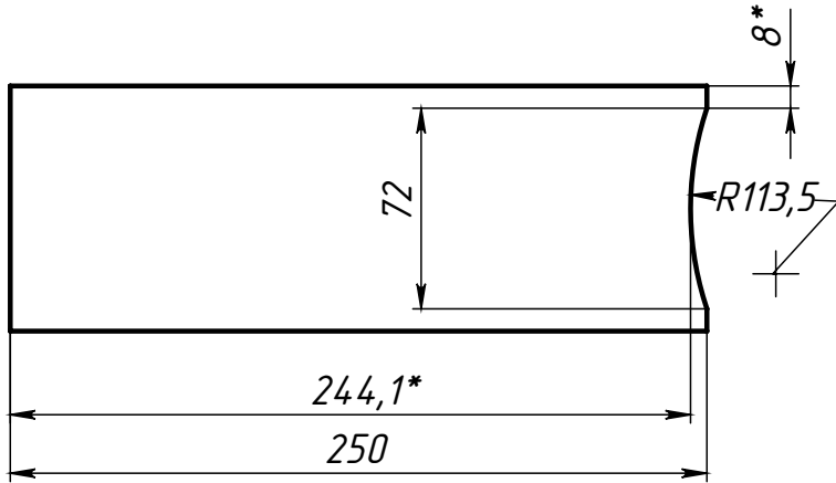
Поз.1 (Основание)
