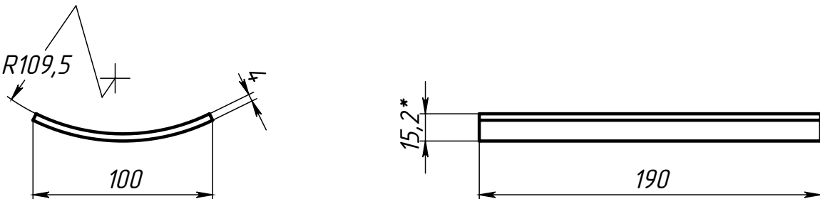
Поз.3 (Ложемент)
